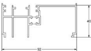
PL258 jamb
