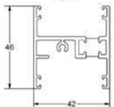
RD11 laybar
